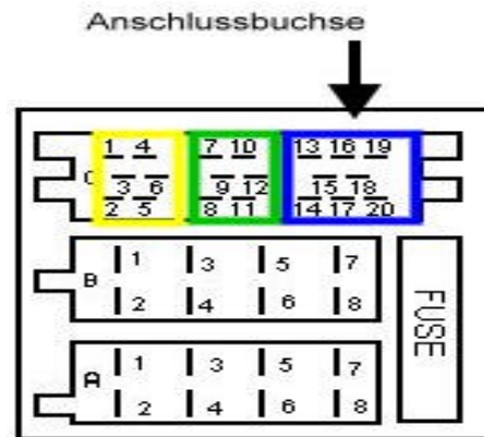
Schema 1
